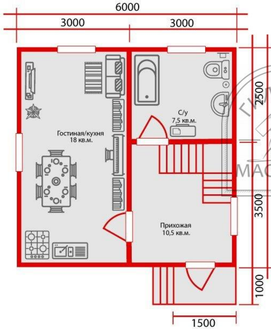
План 1 этажа
