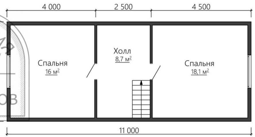
План 2-го этажа
